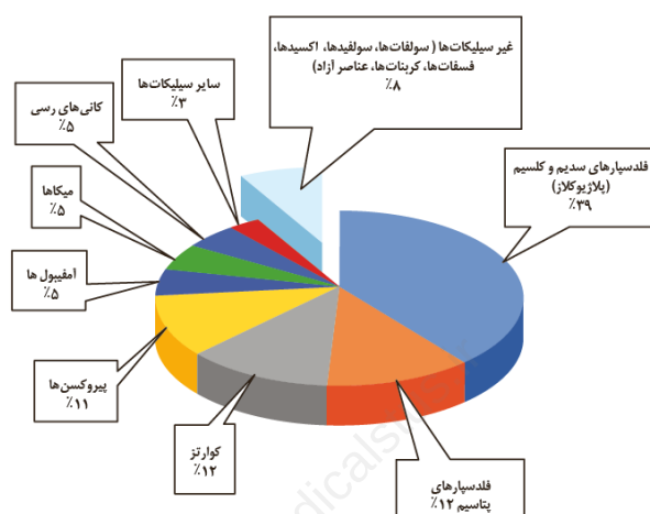
شکل ۳-۲. درصد وزنی کانی های سازنده پوسته زمین
