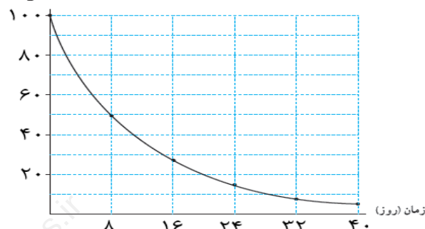
تعداد هسته‌های {}^{131}\text{I}
